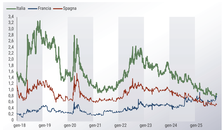
Grafico 27 Spread sovrani: la Spagna meglio della Francia (Titoli a 10 anni, valori, rispetto alla Germania, dati giornalieri)
